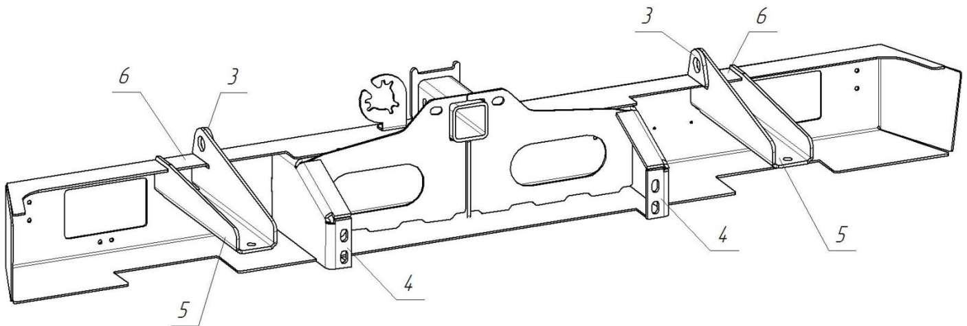
Рис.2 Бампер вид сзади (повёрнут)
