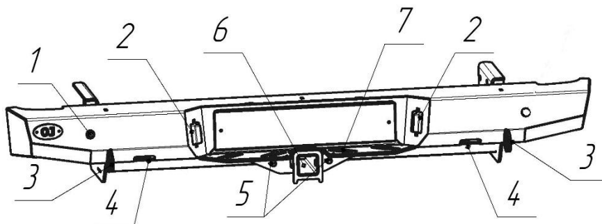
Рис.1 Бампер вид спереди
