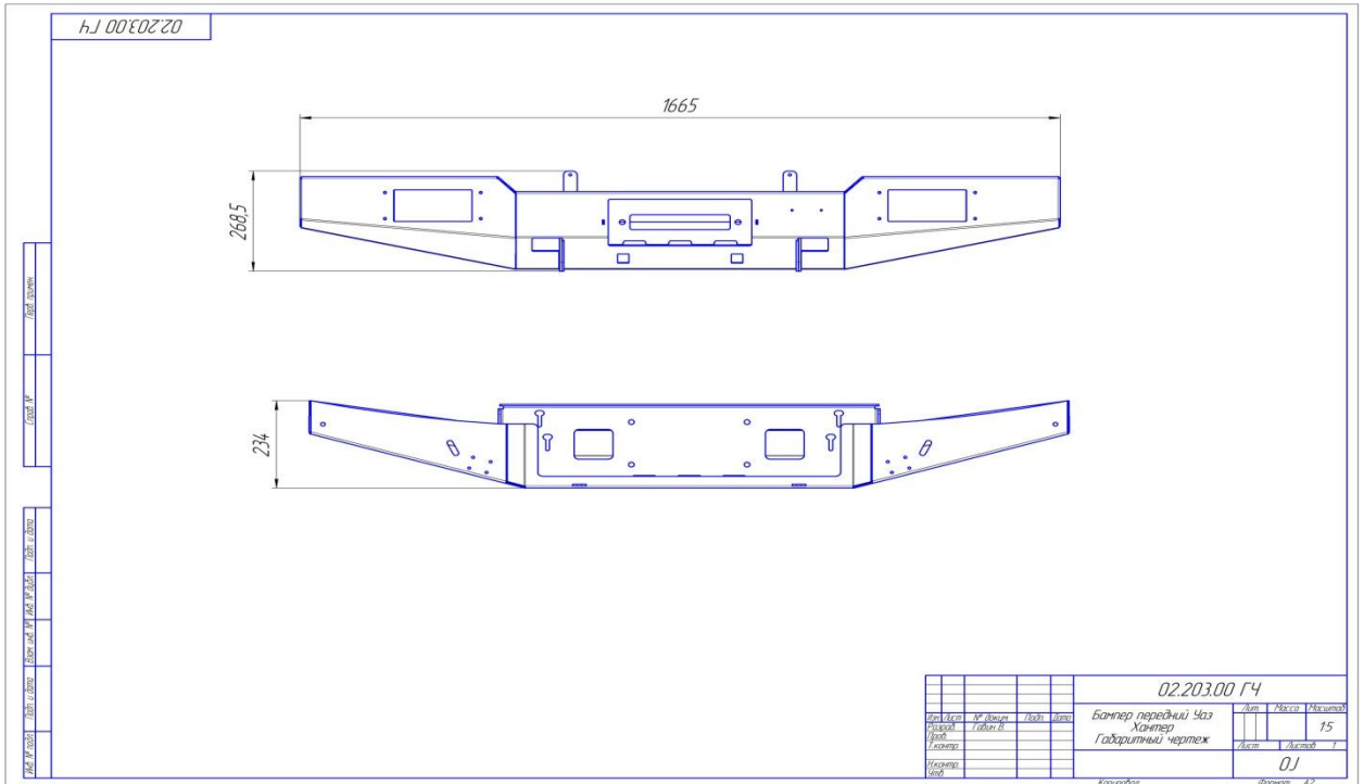
Рис. 3 Габаритный чертёж
