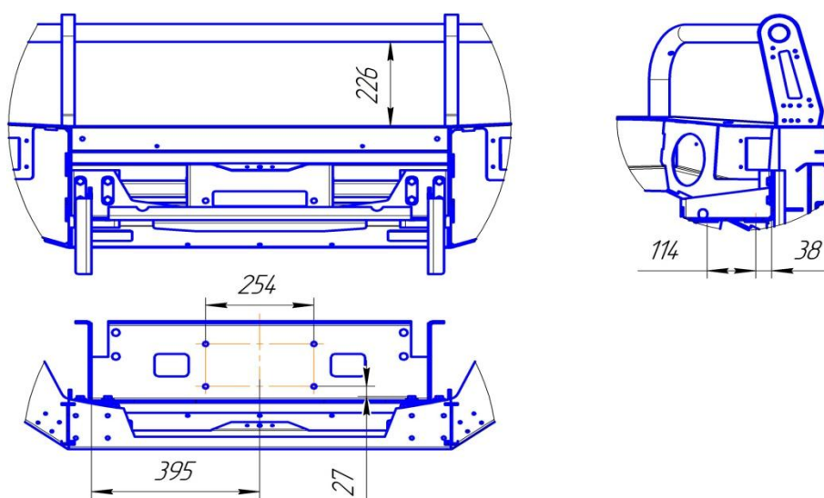
Рис. 4 Габаритный чертёж установки лебедки
