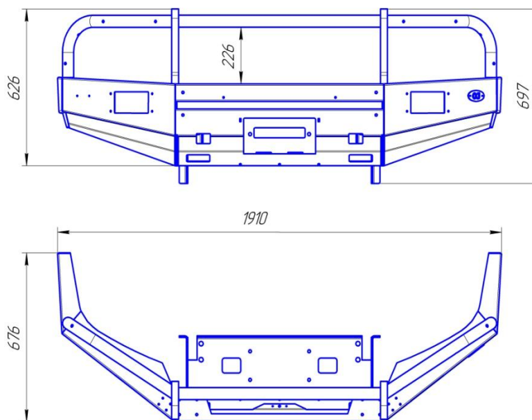
Рис. 3 Габаритный чертёж
