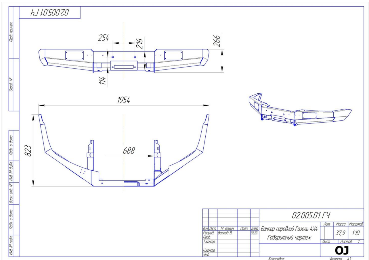
Рис. 3 Габаритный чертёж
