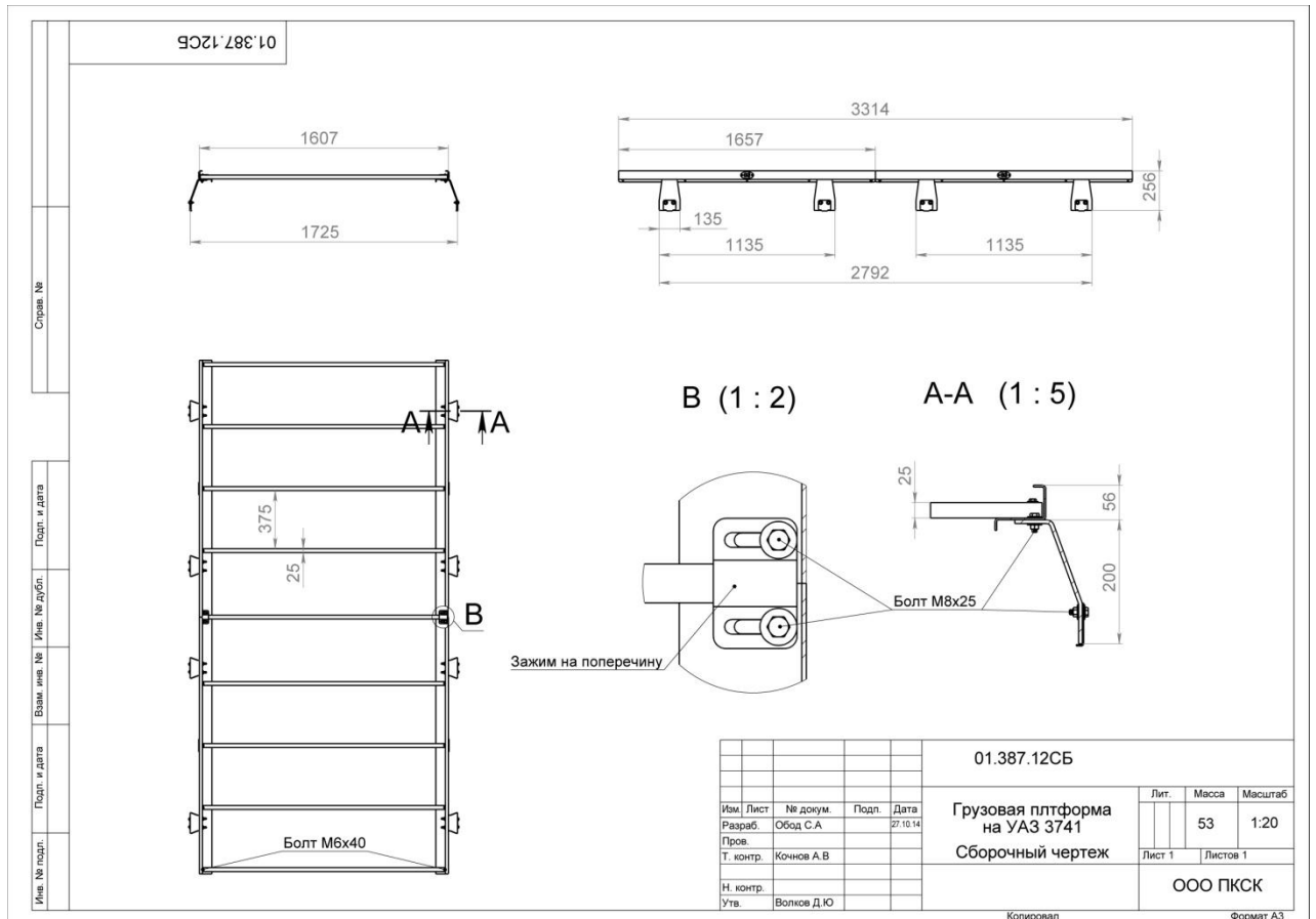
Рис. 2 Сборочный чертёж
