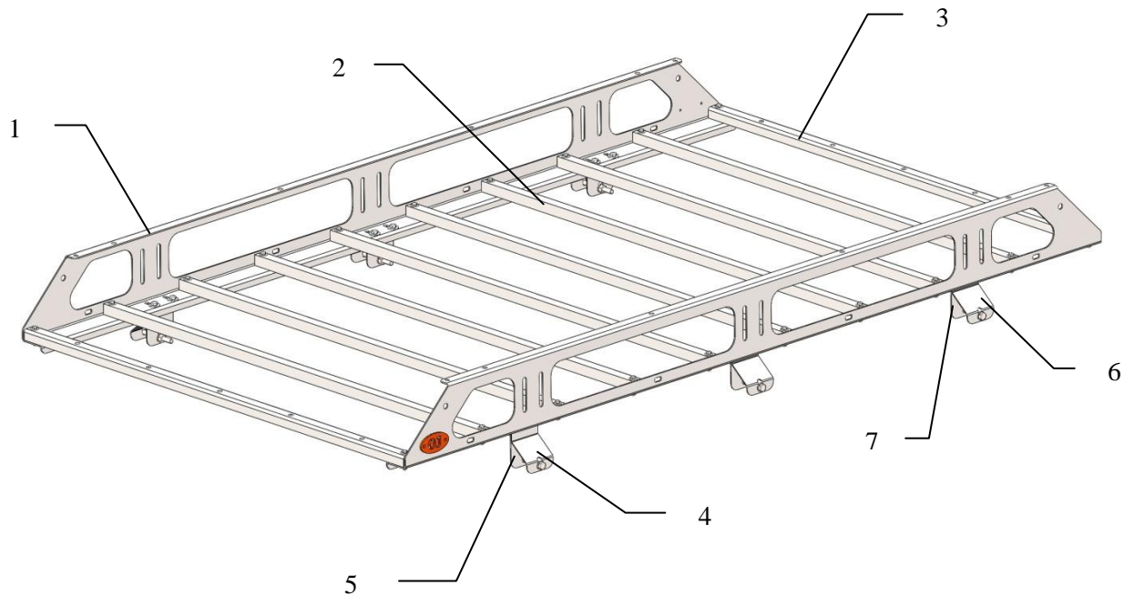
Рис.1 Багажник вид сбоку
