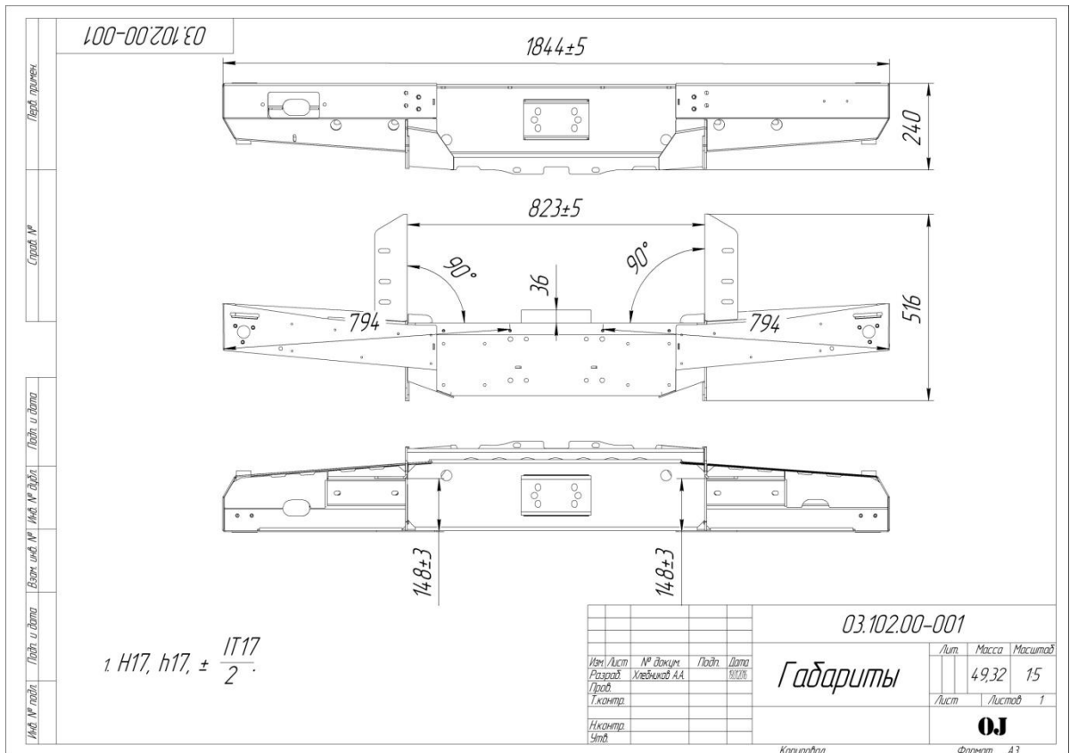
Рис. 3. Габаритный чертёж.
