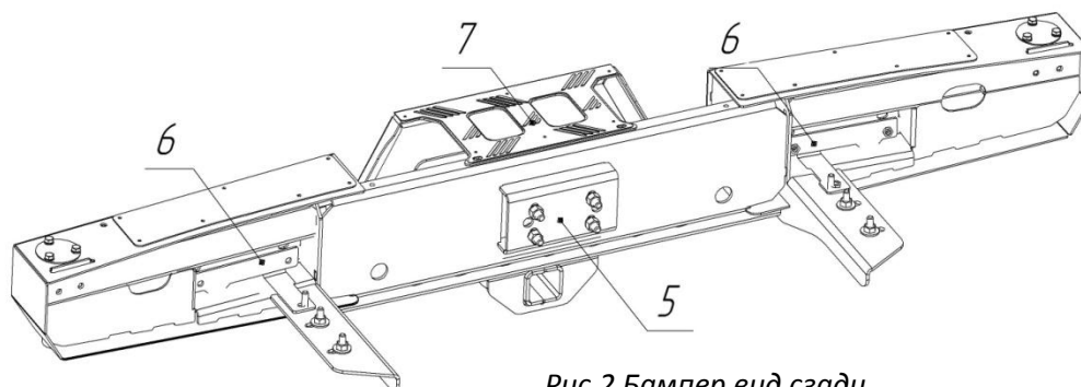
Рис.2 Бампер вид сзади
